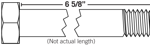
(Not actual length) ADG (x1) 1/2" x 6 5/8" Hex Bolt
